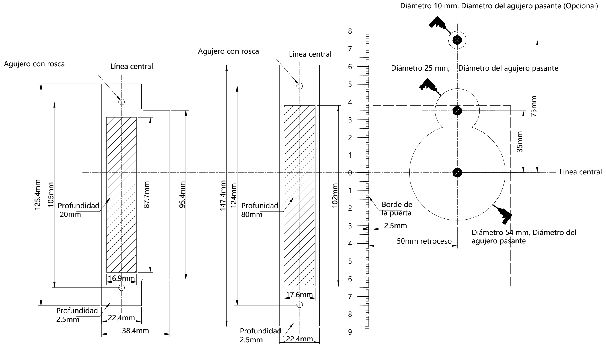
Dibujo técnico del contrafrente
